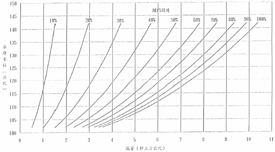
圖四：何本閘開度與放流量關係曲線
