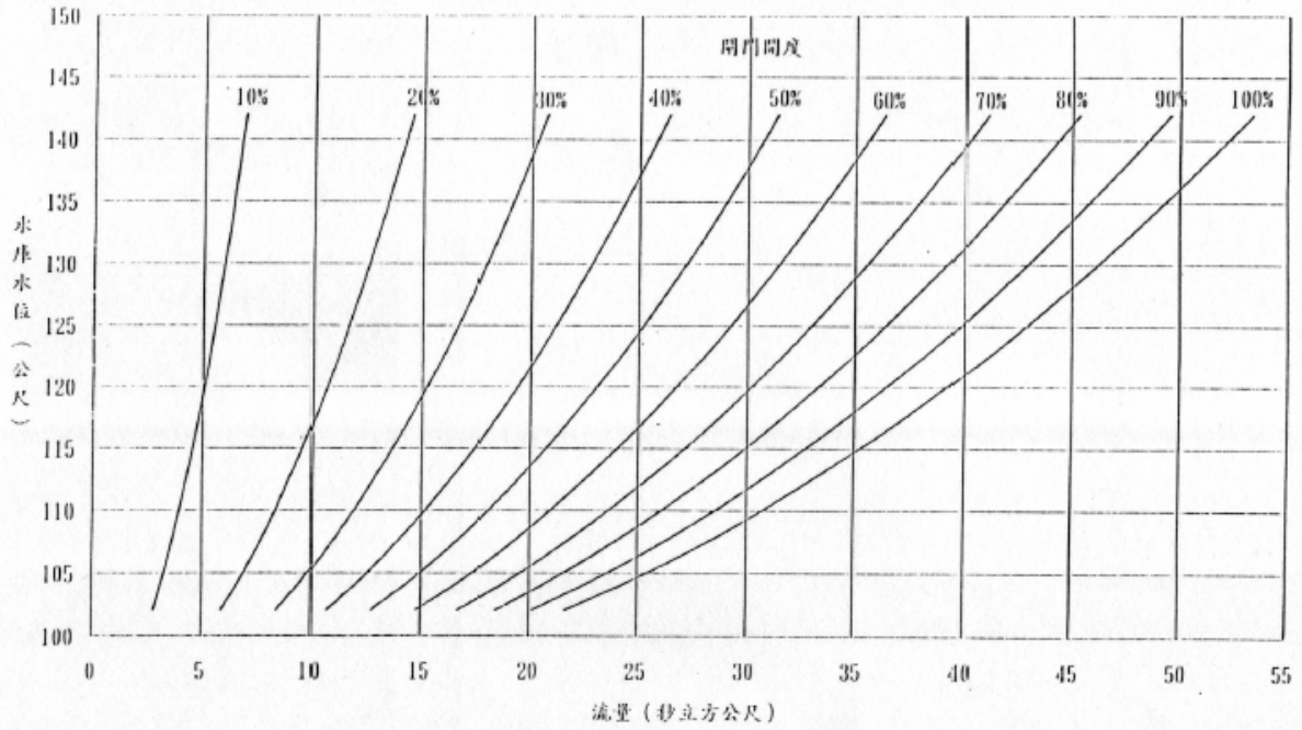
圖三：排水道控制開門開度與放流量關係曲線
