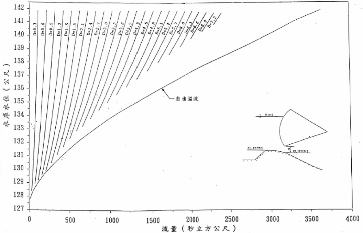
圖二：溢洪道閘門開度與放流量關係曲線（三門）
