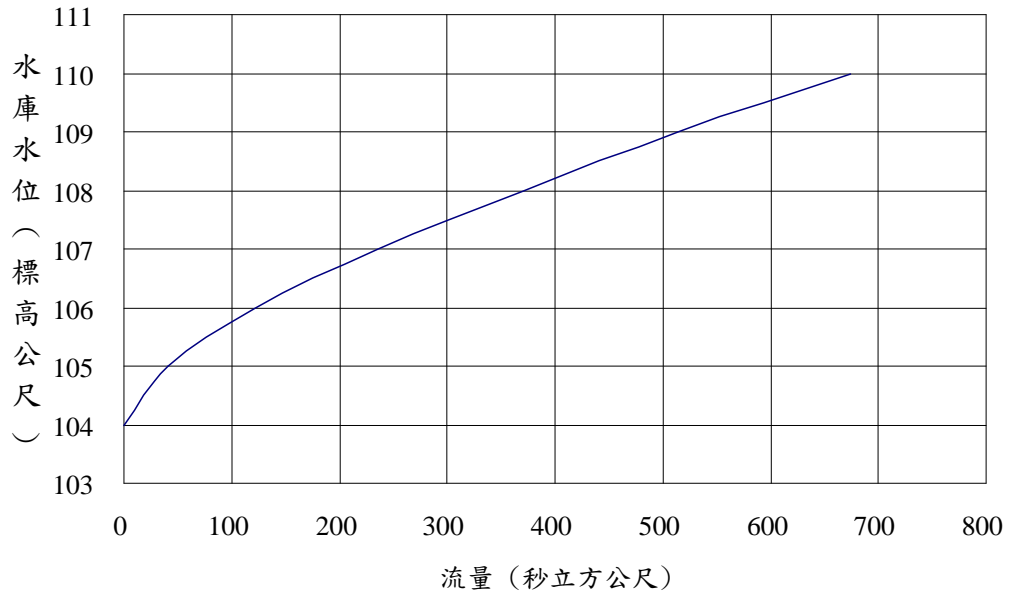
閘門全開率定曲線
